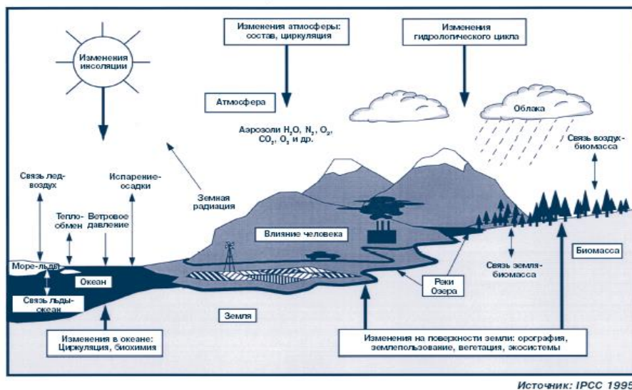
Схематическое изображение климатической системы
